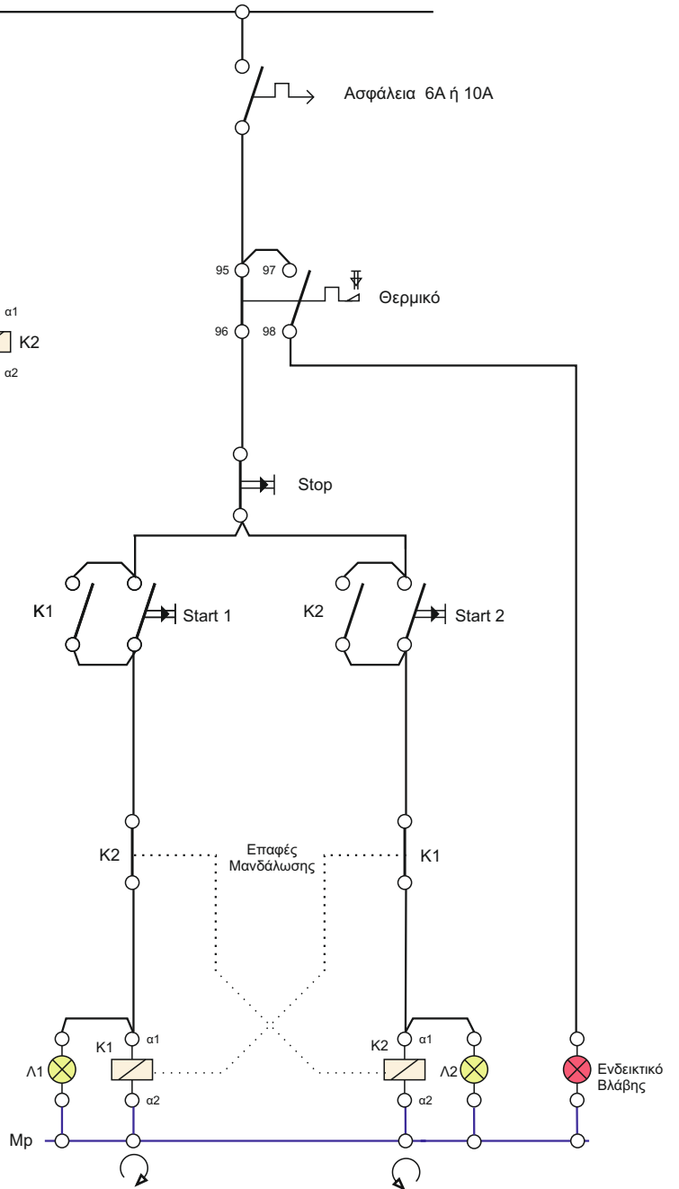
Κύκλωμα Αυτοματισμού
